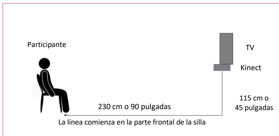
Figura 2: Configuración de Kinect. Vista lateral.
